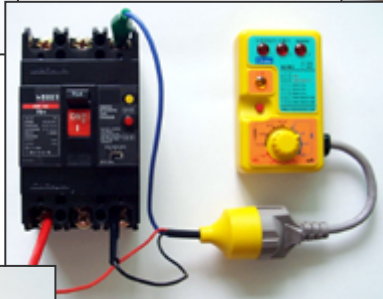
3상누전차단기 시험
