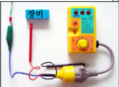
전기장비의 누전확인
